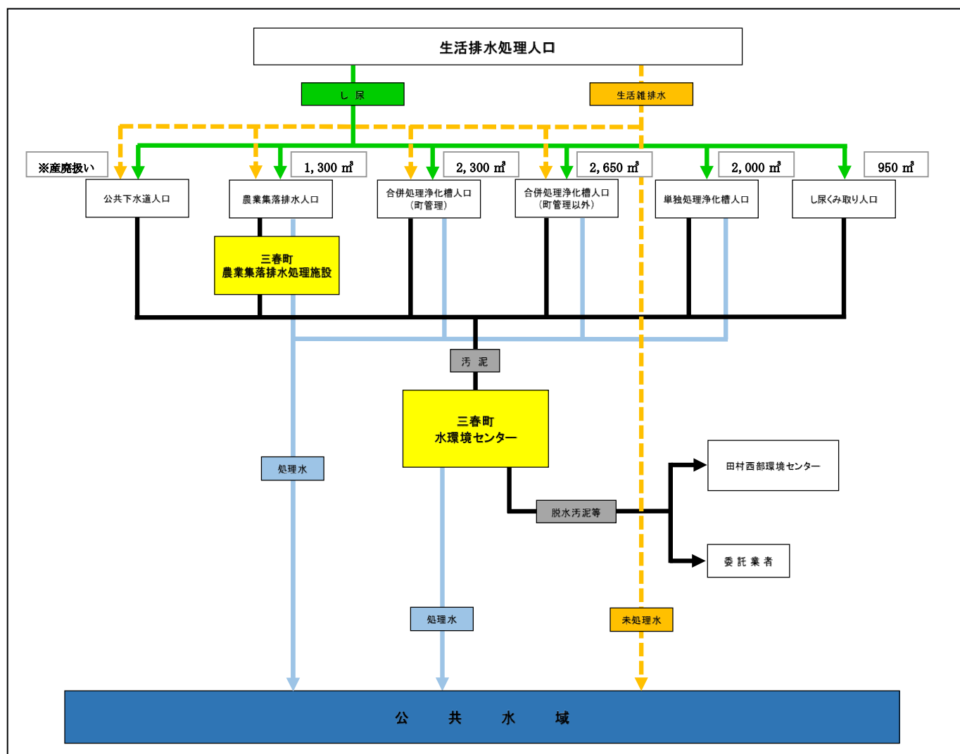
②令和7年度し尿処理計画フロー図
