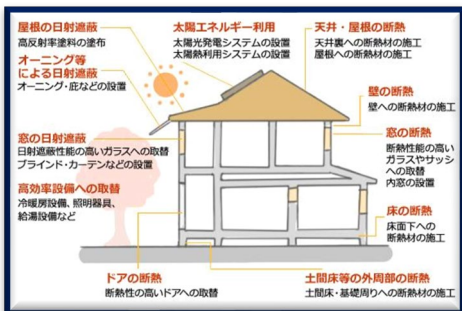
▲省エネリフォームの例 【出典】資源エネルギー庁ウェブサイト
